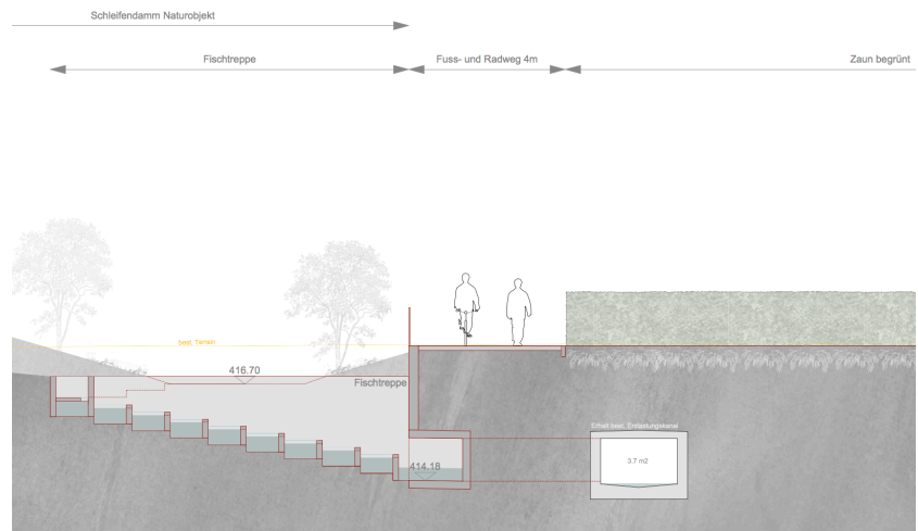
Schnitt Gestaltungsvorschlag Fischtreppe
